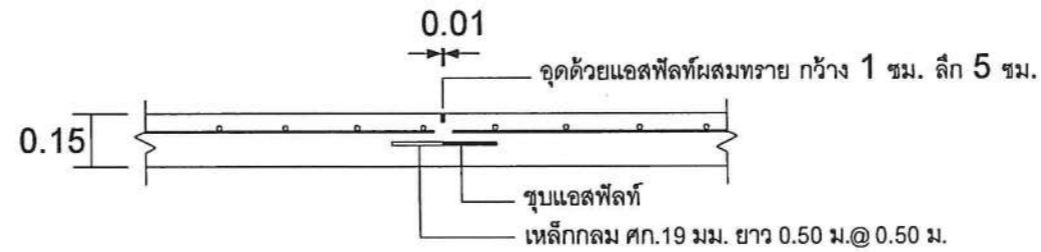
แบบขยาย CONTRACTION JOINT (ใส่ทุกความยาว 5.00 ม.) NOT TO SCALE
