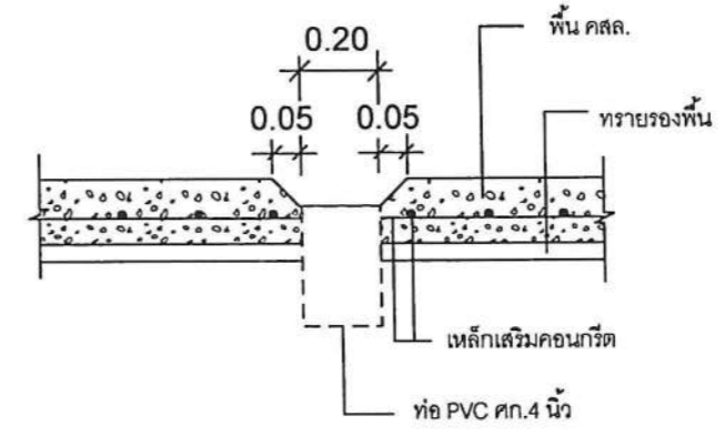
รูปตัดวางระบายน้ำ NOT TO SCALE
