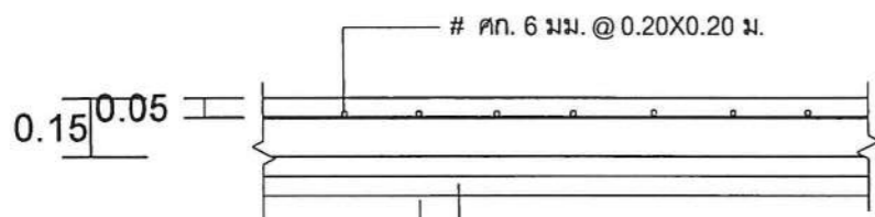
รูปตัด (n)-(n) NOT TO SCALE
