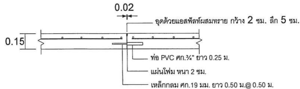
แบบขยาย EXPANSION JOINT (ใส่ทุกความยาว 50.00 ม.) NOT TO SCALE
