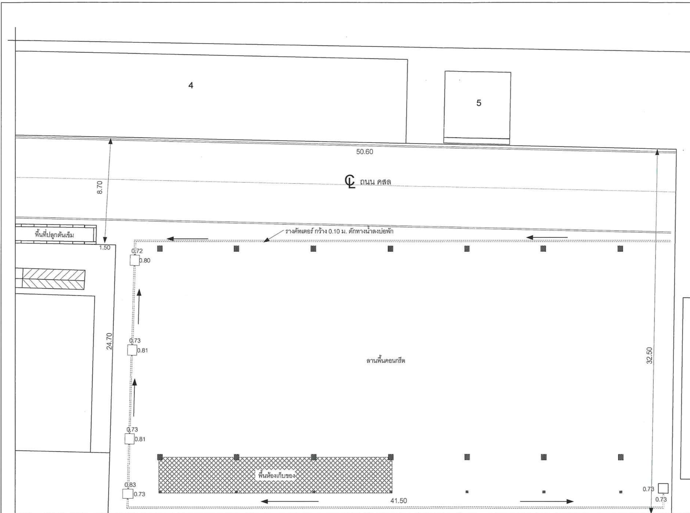
แปลนลานคอนกรีตเสริมเหล็ก NOT TO SCALE
