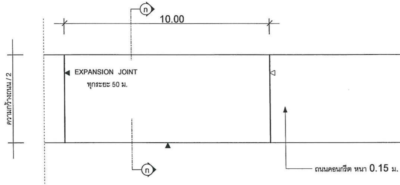
แปลนถนนคอนกรีตเสริมเหล็ก NOT TO SCALE
