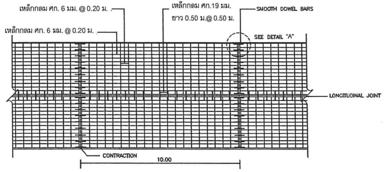
แปลนแสดงการเสริมเหล็ก ถนน NOT TO SCALE
