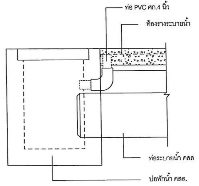
แสดงการต่อท่อ PVC ลงบ่อพักน้ำ NOT TO SCALE
