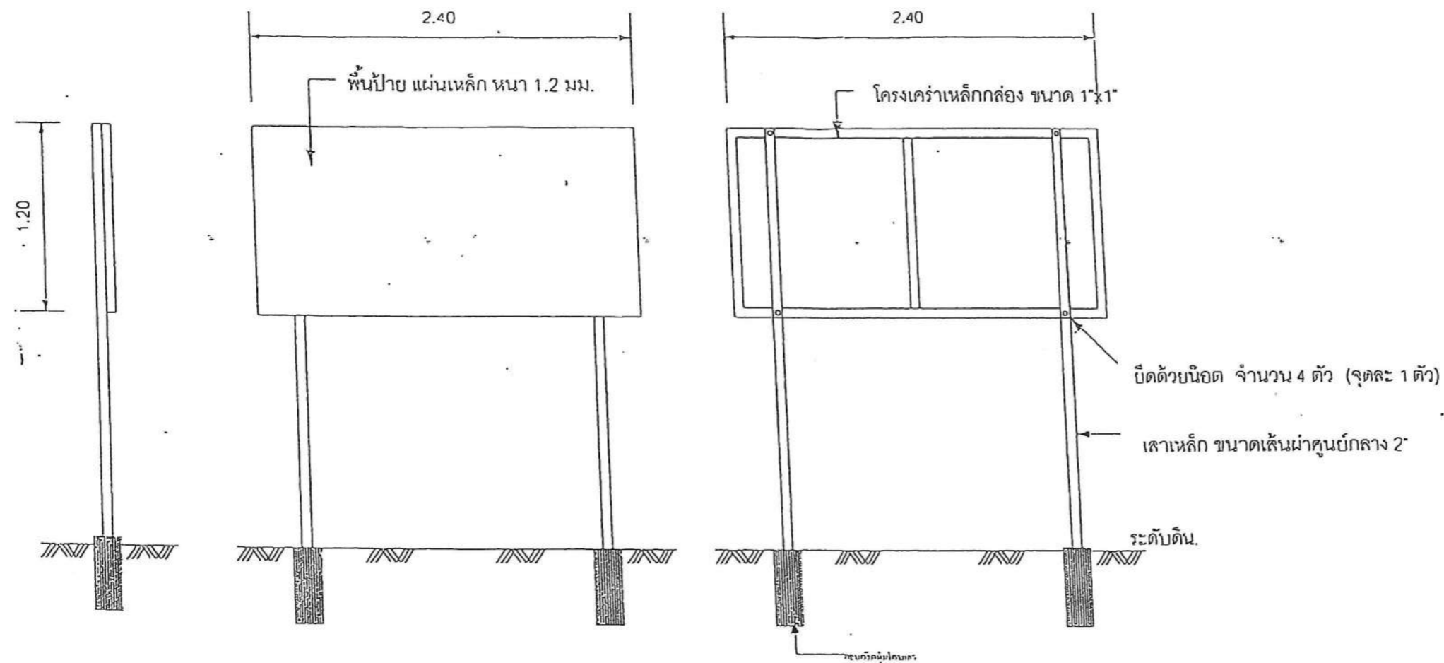
รูปด้านข้าง Non scale
